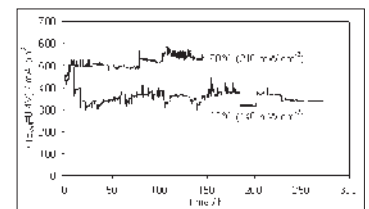
Test di stabilità nel tempo realizzata in una cella \text{H}_2/\text{aria} a 30 e 60^\circ\text{C} .
