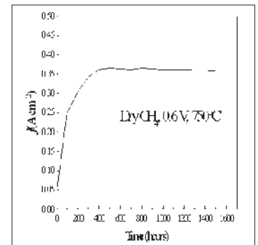
Risultato del test su SOFC Pirelli usando \text{CH}_4 come combustibile.
